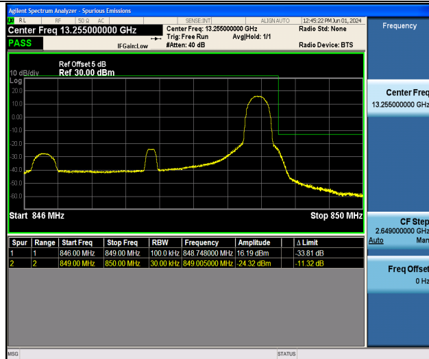
Band5_3MHz_16QAM_20635_1RB#14
