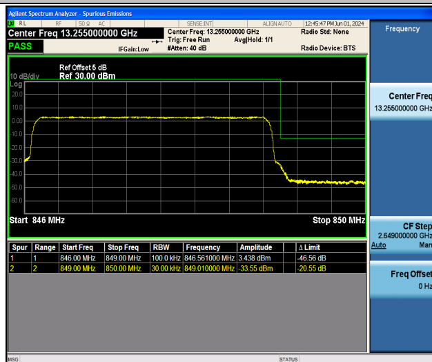
Band5_3MHz_16QAM_20635_15RB#0
