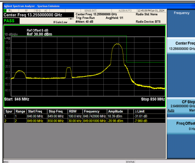
Band5_3MHz_QPSK_20635_1RB#14
