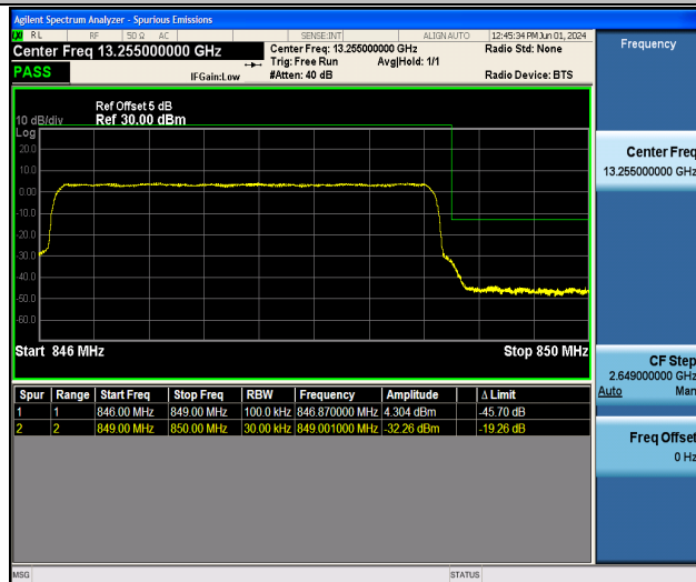
Band5_3MHz_QPSK_20635_15RB#0
