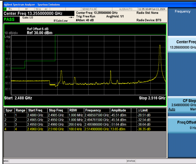
Band41_20MHz_QPSK_39750_1RB#99
