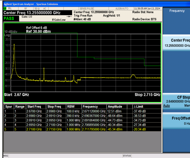
Band41_20MHz_QPSK_41490_1RB#0
