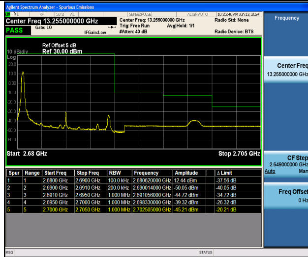
Band41_10MHz_QPSK_41540_1RB#0
