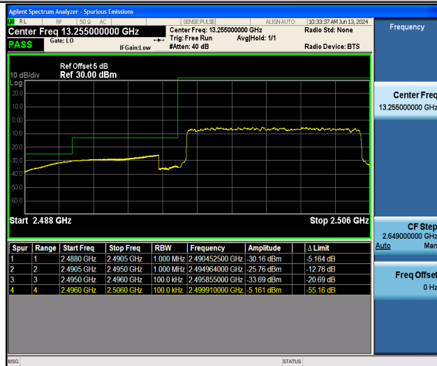
Band41_10MHz_QPSK_39700_50RB#0
