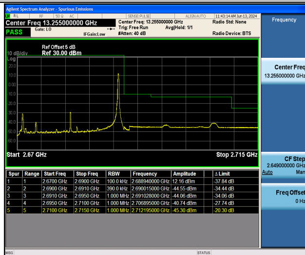
Band41_20MHz_QPSK_41490_1RB#99
