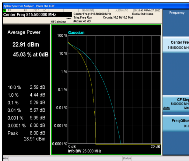
26(814-824)-3MHz-QPSK-26705-15RB#0-PASS
