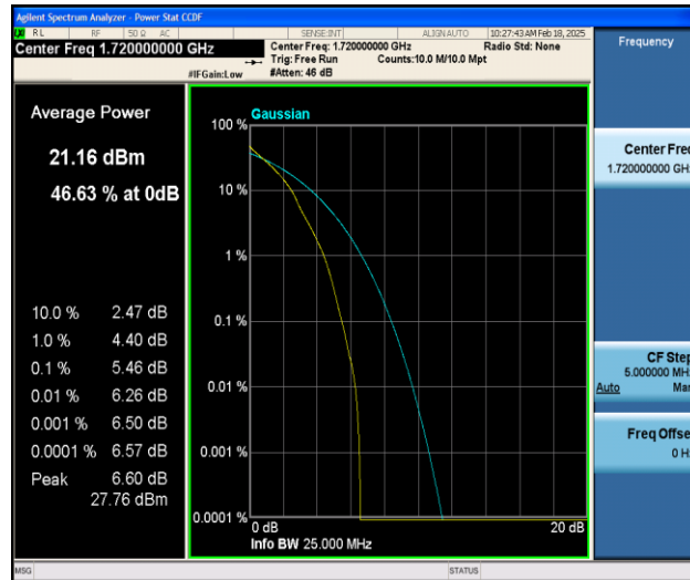
Band66-20MHz-QPSK-132072-1RB#0-PASS
