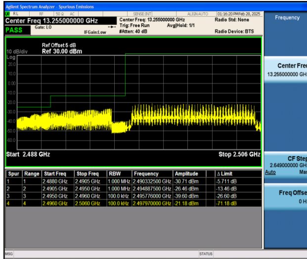
Band41_10MHz_QPSK_39700_50RB#0
