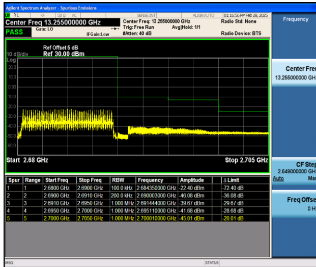
Band41_10MHz_QPSK_41540_50RB#0
