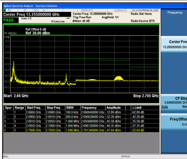
Band41_10MHz_QPSK_41540_1RB#0
