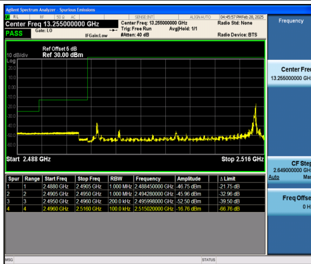
Band41_20MHz_QPSK_39750_1RB#99
