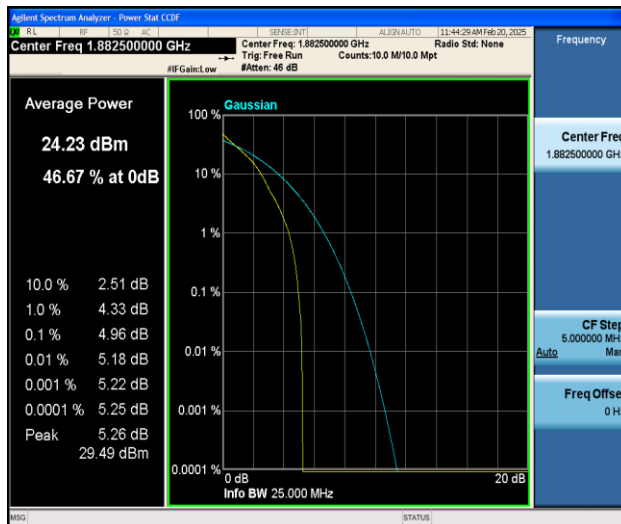
Band25-3MHz-QPSK-26365-1RB#0-PASS
