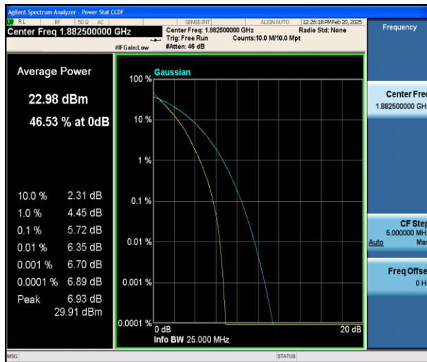
Band25-10MHz-QPSK-26365-50RB#0-PASS
