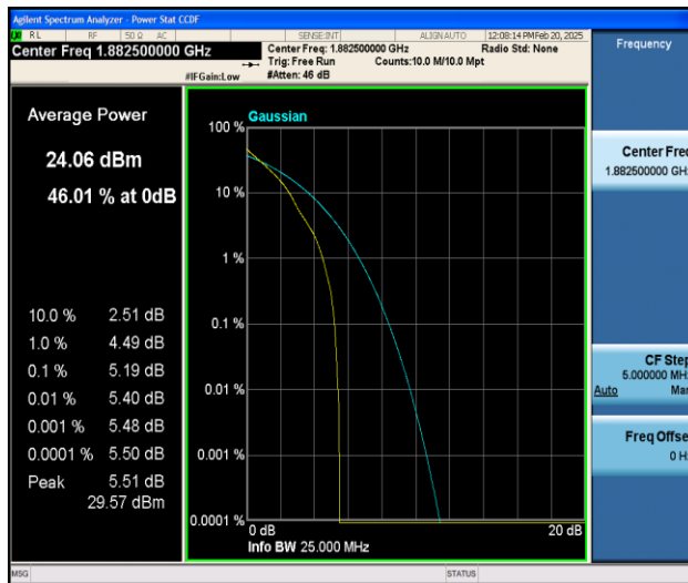
Band25-5MHz-QPSK-26365-1RB#0-PASS
