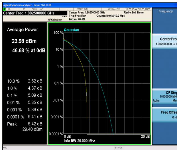
Band25-1.4MHz-QPSK-26365-1RB#0-PASS
