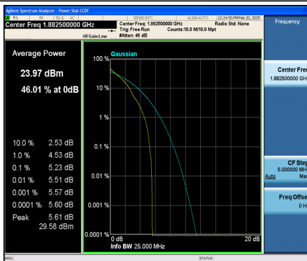
Band25-10MHz-QPSK-26365-1RB#0-PASS
