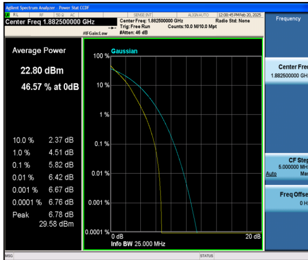
Band25-5MHz-QPSK-26365-25RB#0-PASS
