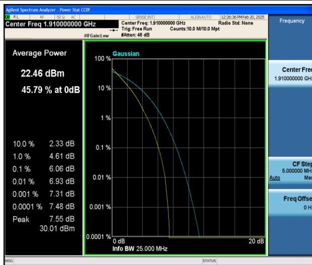
Band25-10MHz-QPSK-26640-50RB#0-PASS
