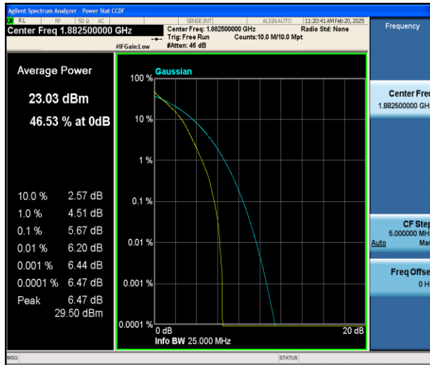
Band25-1.4MHz-QPSK-26365-6RB#0-PASS
