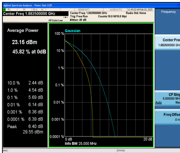
Band25-3MHz-QPSK-26365-15RB#0-PASS
