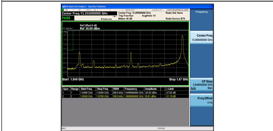
Band2_20MHz_QPSK_18700_1RB#99
