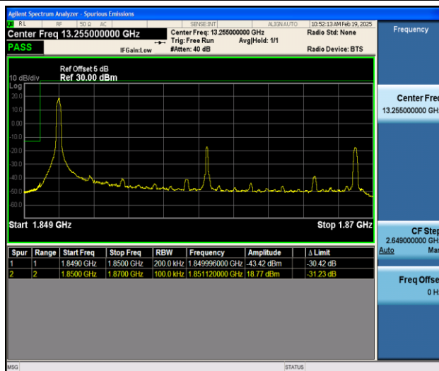
Band2_20MHz_QPSK_18700_1RB#0
