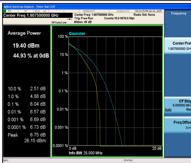
Band2-5MHz-QPSK-19175-1RB#0-PASS
