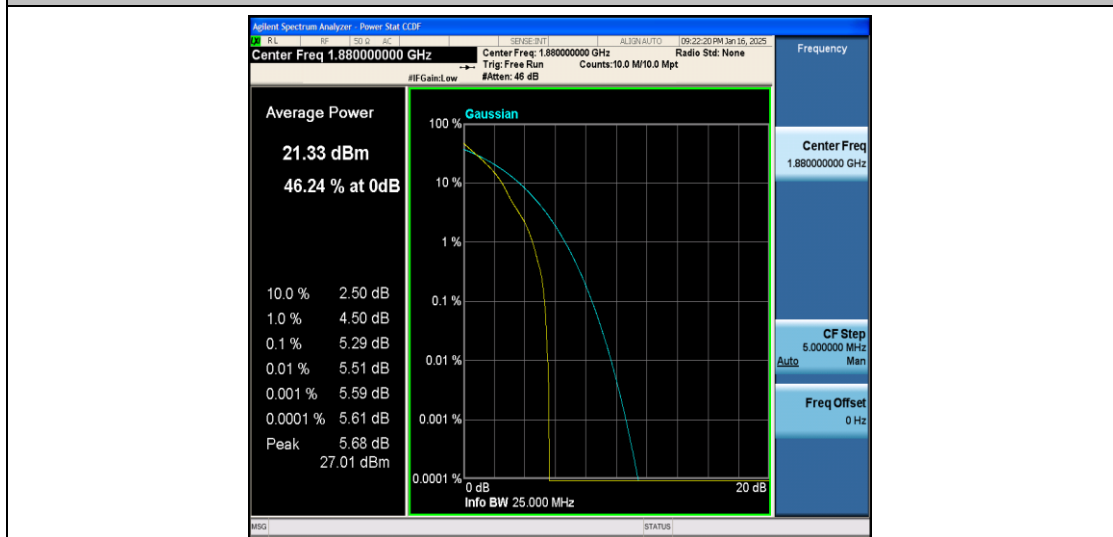
Band2-5MHz-QPSK-18900-1RB#0-PASS
