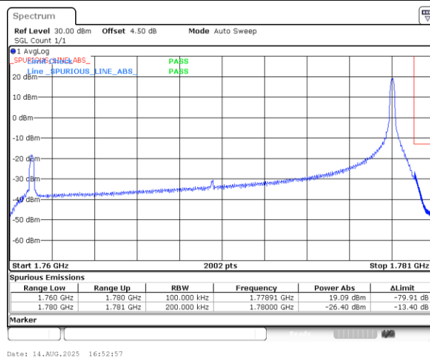
Band66_20MHz_QPSK_132572_1RB#99
