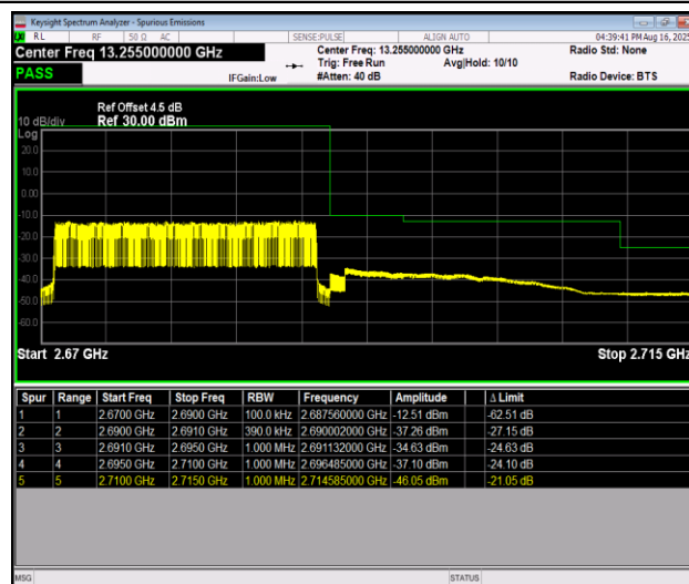
Band41_20MHz_QPSK_41490_100RB#0
