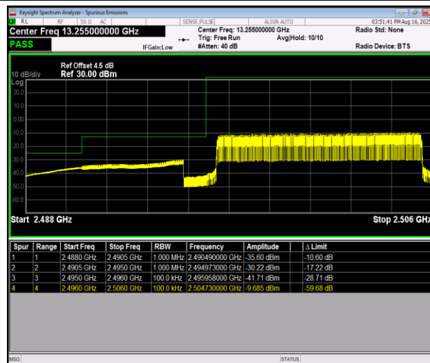
Band41_10MHz_QPSK_39700_50RB#0
