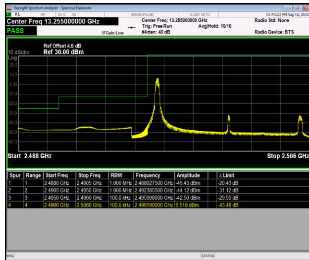
Band41_10MHz_QPSK_39700_1RB#0
