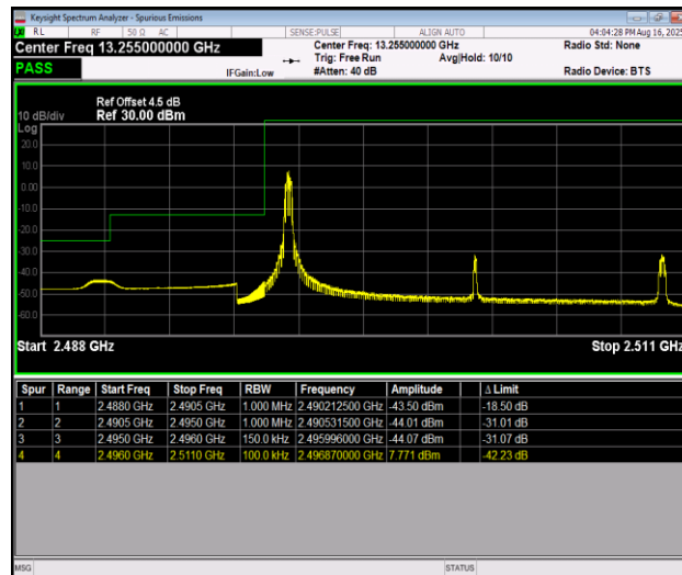
Band41_15MHz_QPSK_39725_1RB#0
