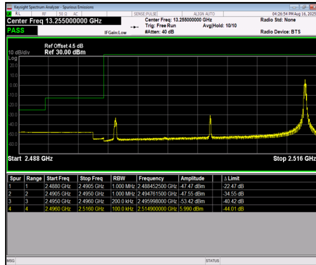
Band41_20MHz_QPSK_39750_1RB#99
