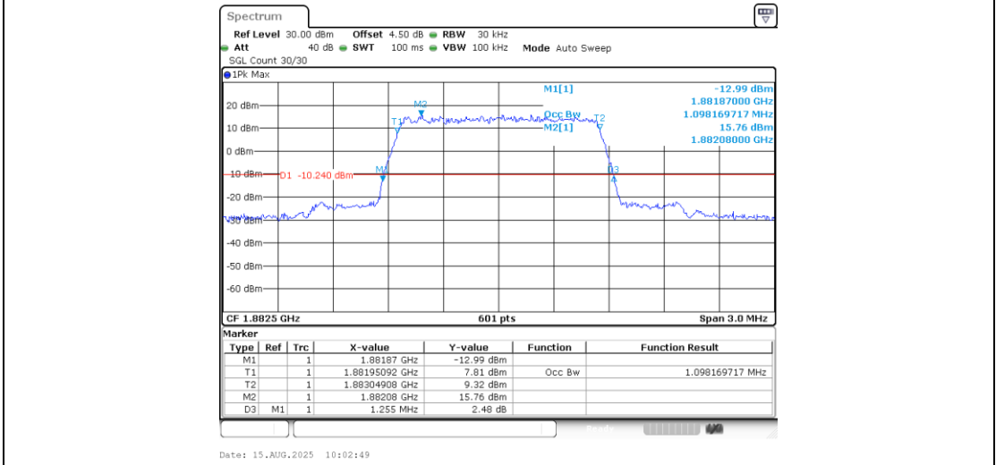
Band25-1.4MHz-QPSK-26365-6RB#0-PASS
