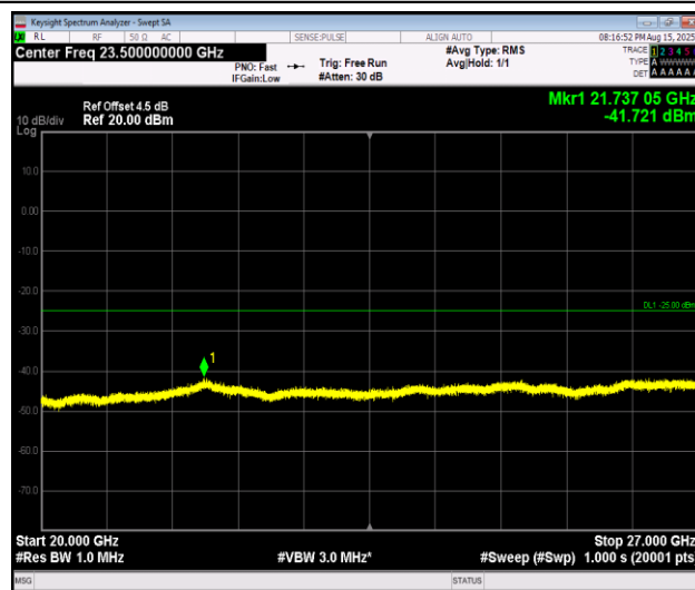
Band7_20MHz_QPSK_20850_1RB#0_20000~27000_20000~27000
