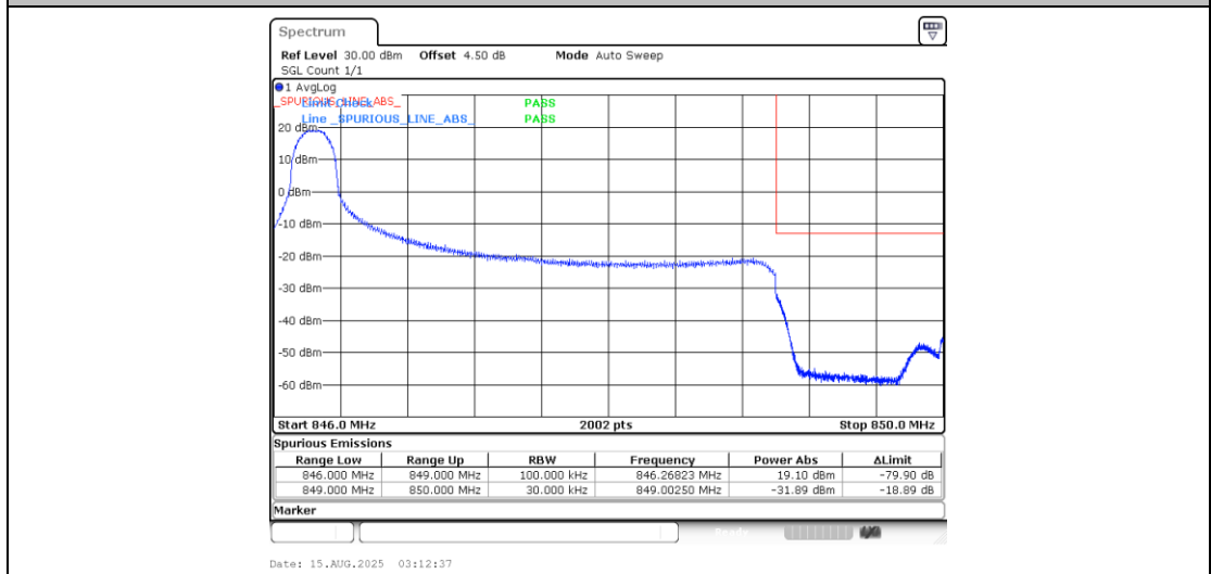
Band5_3MHz_16QAM_20635_1RB#0
