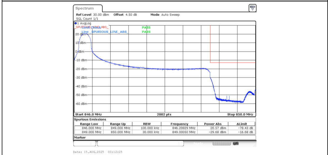
Band5_3MHz_QPSK_20635_1RB#0
