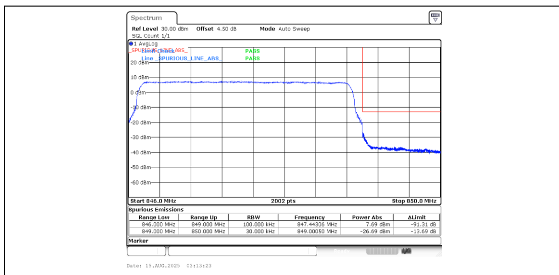
Band5_3MHz_16QAM_20635_15RB#0
