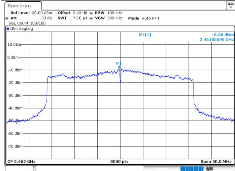
PSD NVNT ax20 2462MHz Ant1
