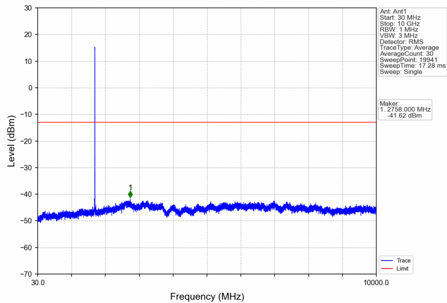
Band4_HSUPA_LCH_1712.4MHz_Subtest 1_NTNV
