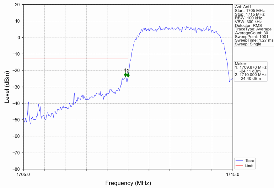
Band4_HSUPA_LCH_1712.4MHz_Subtest 1_NTNV
