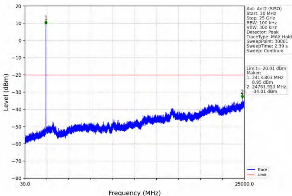
802.11b_LCH_2412MHz_Ant2 (SISO)_NTNV
