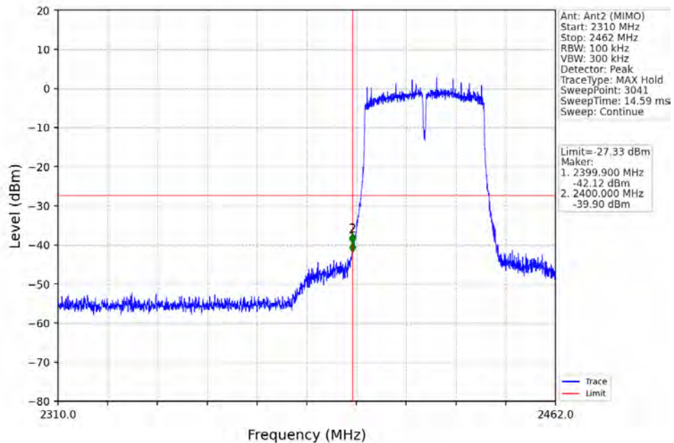
802.11n(HT40)_LCH_2422MHz_Ant2 (MIMO)_NTNV
