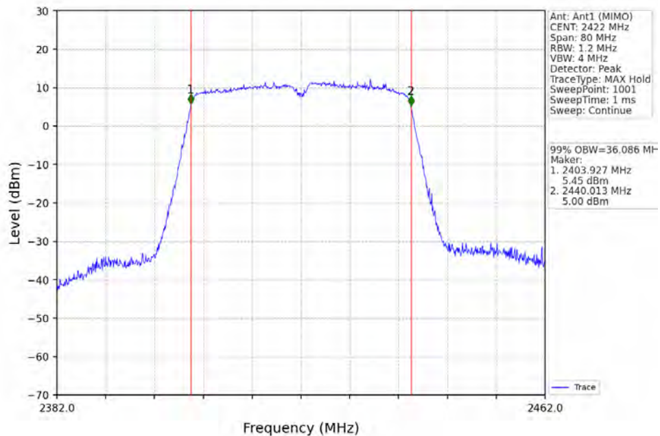
802.11n(HT40)_LCH_2422MHz_Ant1 (MIMO)_NTNV
