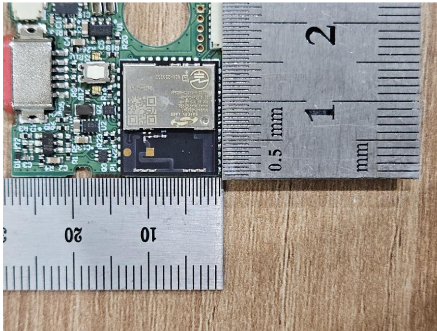
Bluetooth Module
