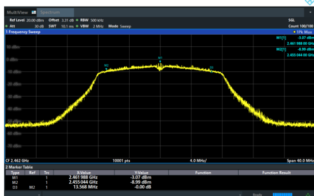
TX CH 11
