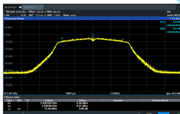
TX CH 06
