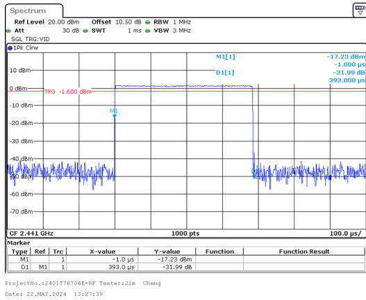
GFSK_Hopping_DH1 0.393ms
