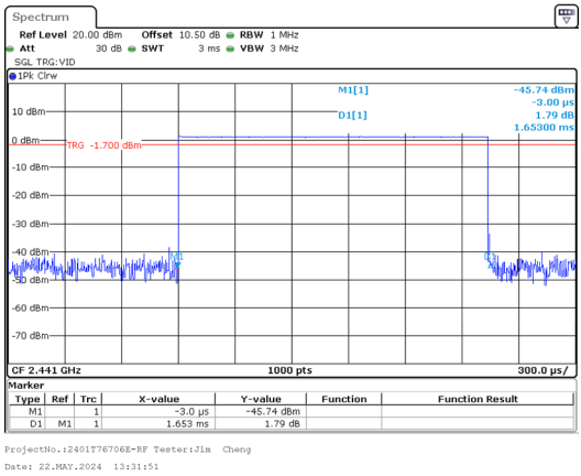
GFSK_Hopping_DH3 1.653ms
