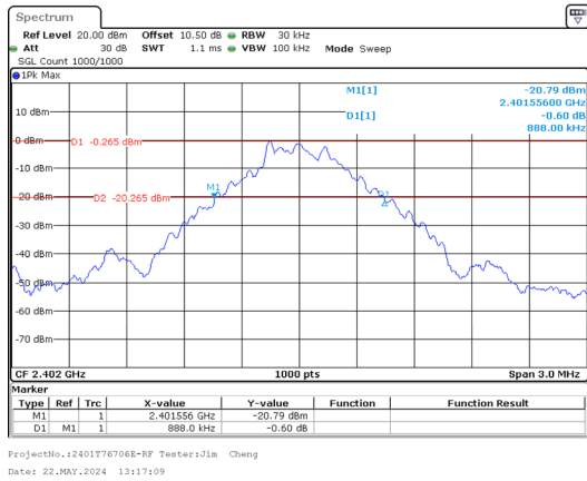
GFSK_Low 0.888MHz
