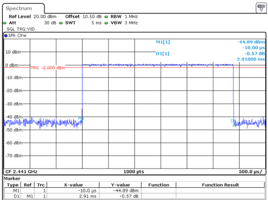
\pi/4 -DQPSK_Hopping_2DH5 2.910ms
