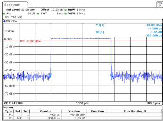
GFSK_Hopping_DH1 0.388ms
