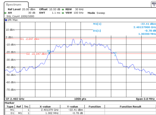
\pi/4 -DQPSK_Low 1.302MHz
