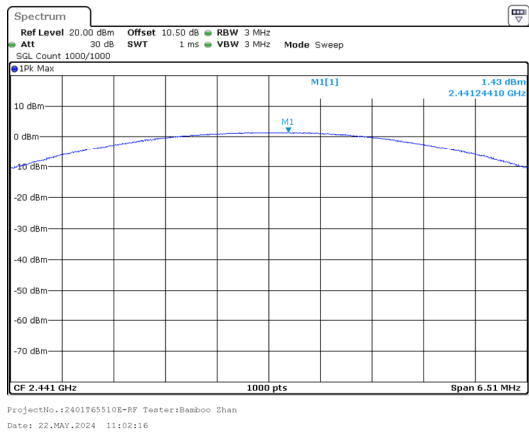
\pi/4 -DQPSK_Middle 1.43dBm
