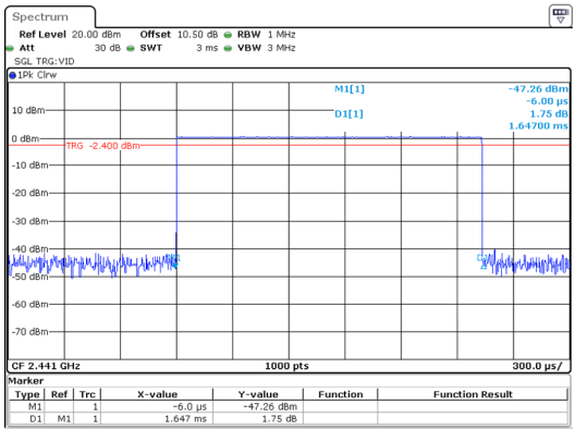
GFSK_Hopping_DH3 1.647ms
