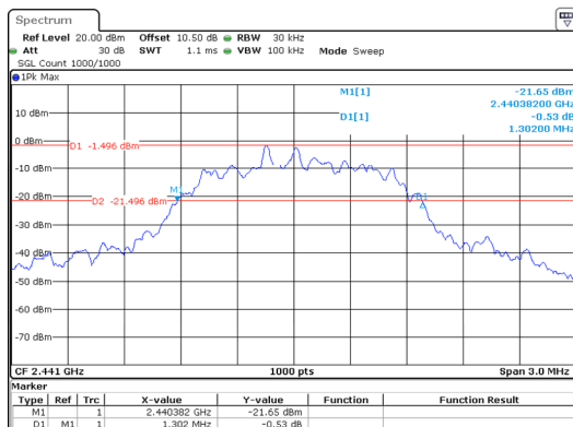
\pi/4 -DQPSK_Middle 1.302MHz
