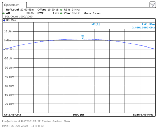
\pi/4 -DQPSK_High 1.61dBm
