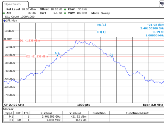
GFSK_Low 1.008MHz
