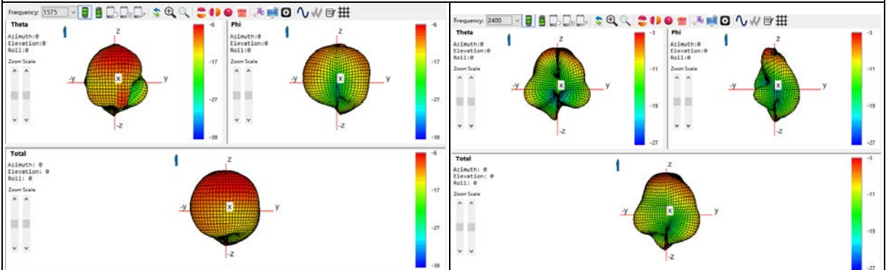
GPS/BT:1575Mhz
