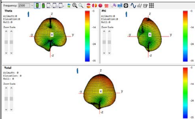
GPS/BT: 2500Mhz
