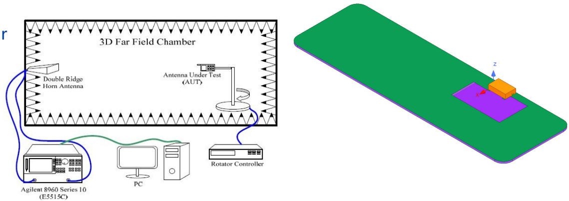
Fig.2 暗室示意图
