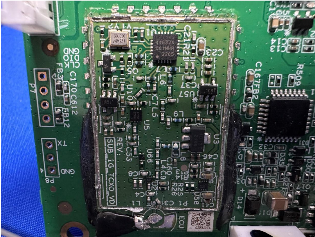
(9) EUT Photo
