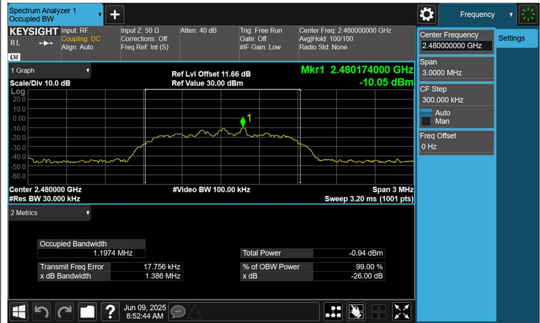
2DH5_Ant1_2480
