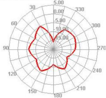
2500.000MHz H
