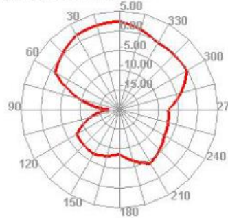
2450.000MHz E1
