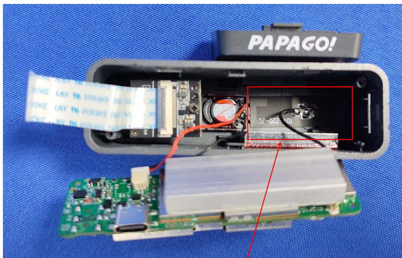
Antenna
