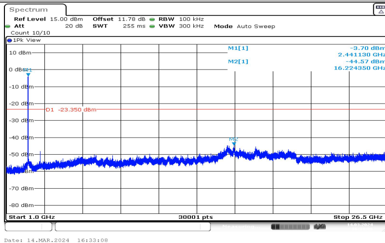
11G-Ant1-2437-1000~26500--3.35
