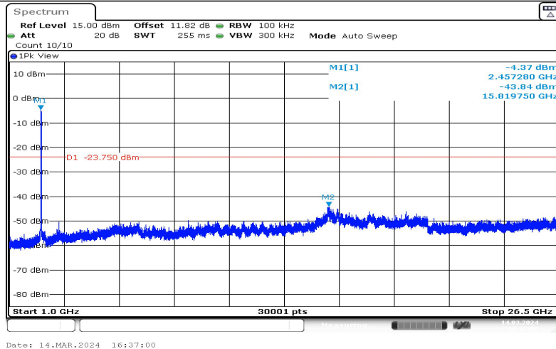
11G-Ant1-2462-1000~26500--3.75
