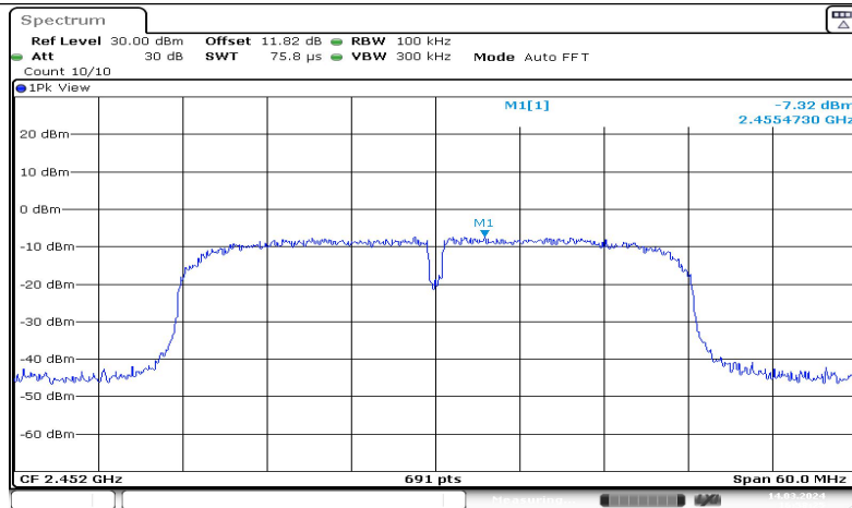
11N40SISO-Ant1-2452-0~Reference--7.32
