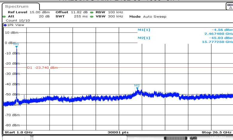
11N20SISO-Ant1-2462-30~1000--3.74
