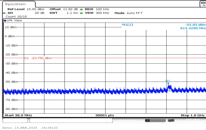
11G-Ant1-2462-30~1000--3.75
