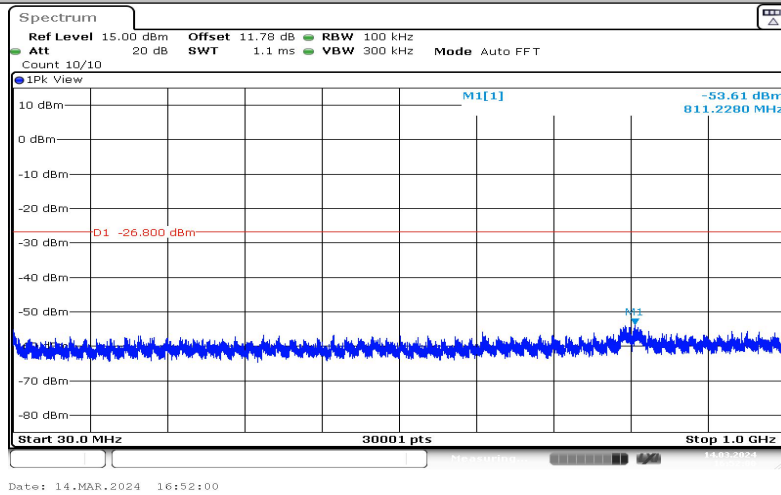
11N40SISO-Ant1-2422-30~1000--6.80
