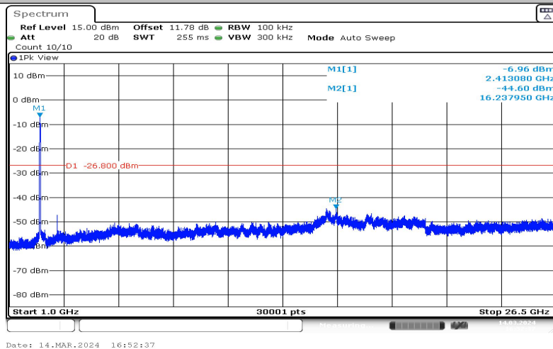
11N40SISO-Ant1-2422-1000~26500--6.80
