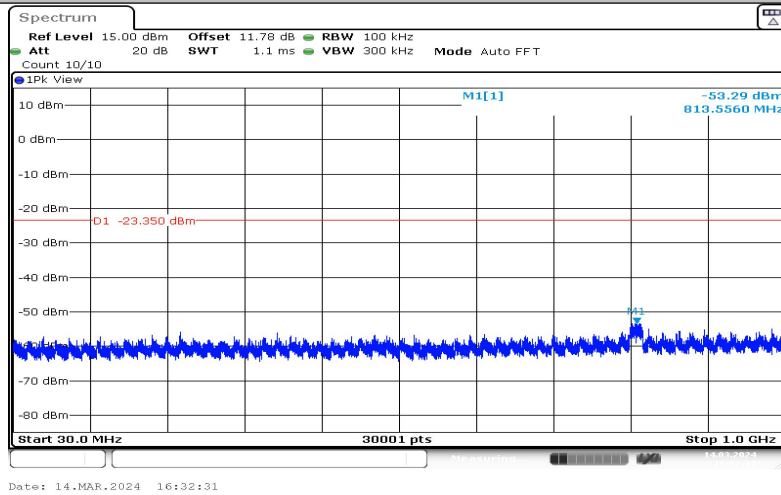
11G-Ant1-2437-30~1000--3.35
