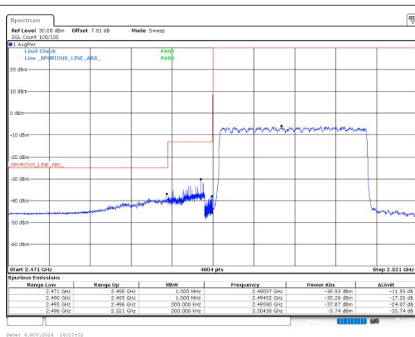
n41 SCS=30kHz DFT_256QAM BW=20MHz LowChannel=501204 RB=50@0
