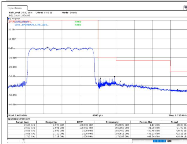
n41 SCS=30kHz DFT_16QAM BW=20MHz HighChannel=535998 RB=50@0
