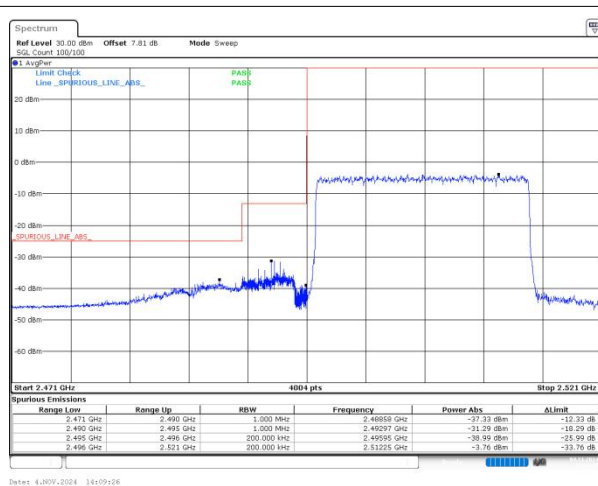
n41 SCS=30kHz DFT_64QAM BW=20MHz LowChannel=501204 RB=50@0
