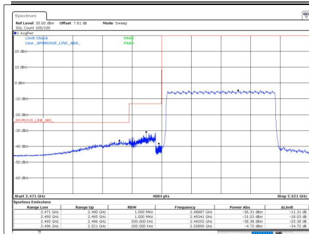
n41 SCS=30kHz CP_QPSK BW=20MHz LowChannel=501204 RB=51@0
