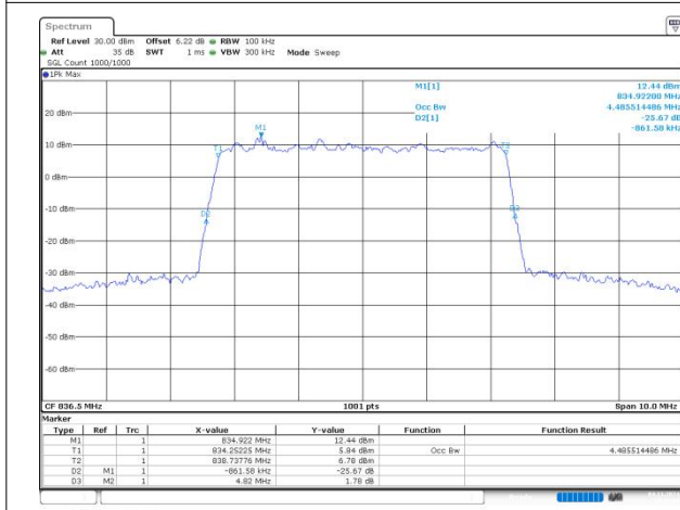
n26(824-849) SCS=15kHz CP_16QAM BW=5MHz Channel=167300 RB=25@0
