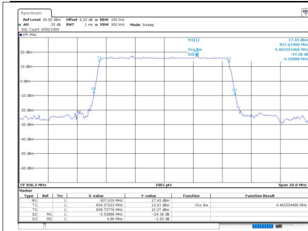
n26(824-849) SCS=15kHz DFT_BPSK BW=5MHz Channel=167300 RB=25@0
