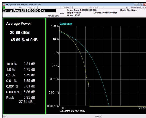
n25 SCS=15kHz DFT_64QAM BW=20MHz Channel=376500 RB=100@0
