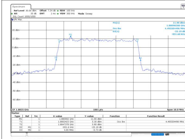
n25 SCS=15kHz CP_256QAM BW=5MHz Channel=376500 RB=25@0
