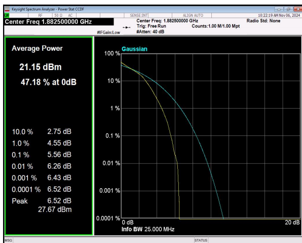
n25 SCS=15kHz DFT_16QAM BW=20MHz Channel=376500 RB=100@0
