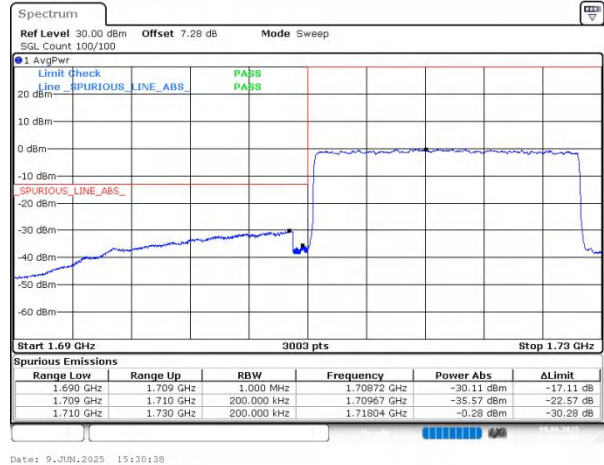
n66 SCS=15kHz DFT_256QAM BW=20MHz LowChannel=344000 RB=100@0
