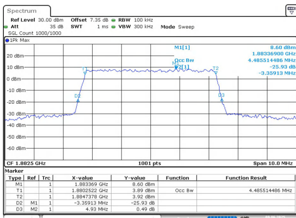
n25 SCS=15kHz CP_16QAM BW=5MHz Channel=376500 RB=25@0
