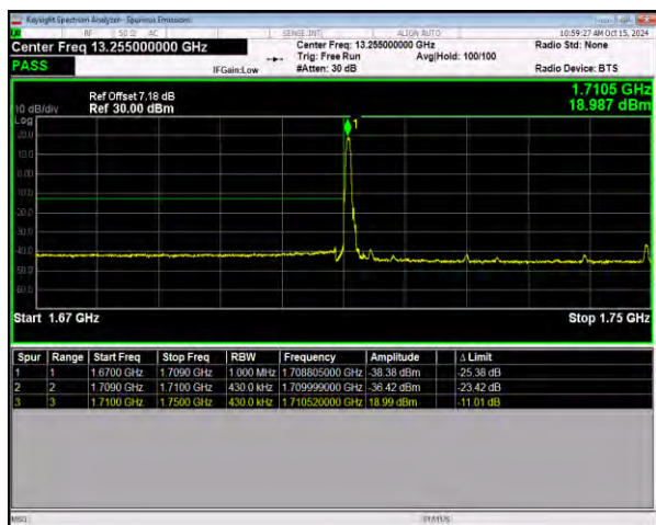
n66 SCS=15kHz DFT_256QAM BW=40MHz
