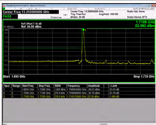
n66 SCS=15kHz DFT_BPSK BW=25MHz LowChannel=344500
