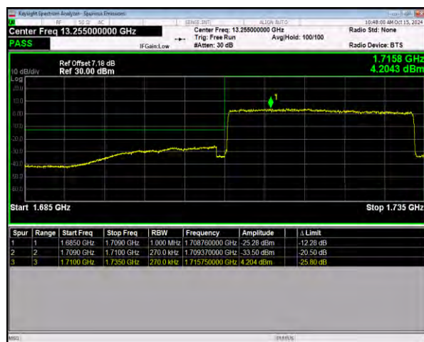
n66 SCS=15kHz DFT_QPSK BW=25MHz LowChannel=344500 RB=128@0
