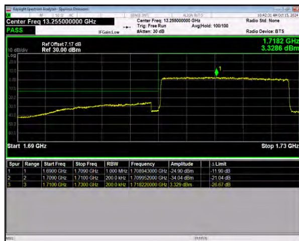
n66 SCS=15kHz DFT_QPSK BW=20MHz LowChannel=344000 RB=100@0
