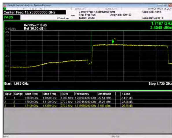
n66 SCS=15kHz DFT_16QAM BW=25MHz LowChannel=344500 RB=128@0
