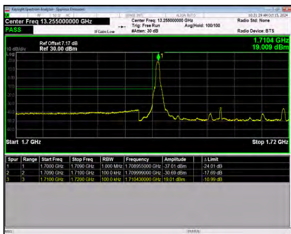
n66 SCS=15kHz DFT_QPSK BW=10MHz LowChannel=343000 RB=1@0
