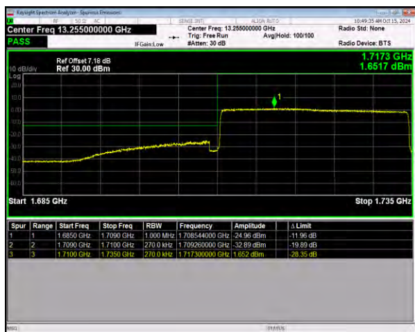
n66 SCS=15kHz CP_QPSK BW=25MHz LowChannel=344500
