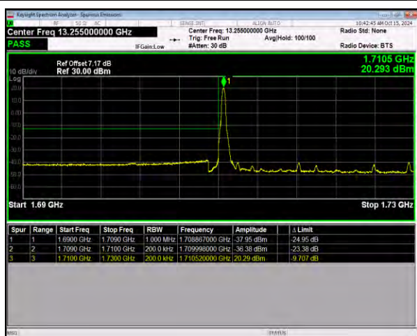
n66 SCS=15kHz DFT_16QAM BW=20MHz LowChannel=344000 RB=1@0
