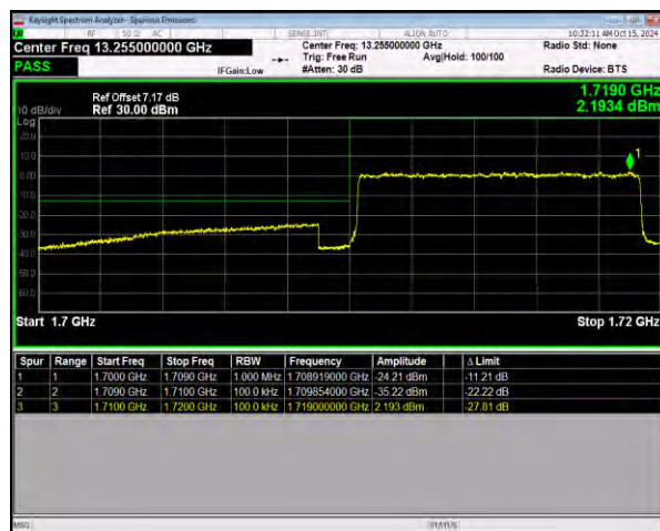
n66 SCS=15kHz DFT_16QAM BW=10MHz LowChannel=343000 RB=50@0
