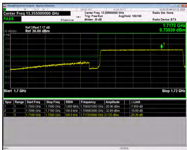
n66 SCS=15kHz CP_QPSK BW=10MHz LowChannel=343000
