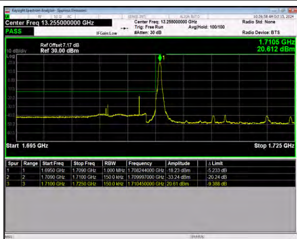
n66 SCS=15kHz DFT_QPSK BW=15MHz LowChannel=343500 RB=1@0
