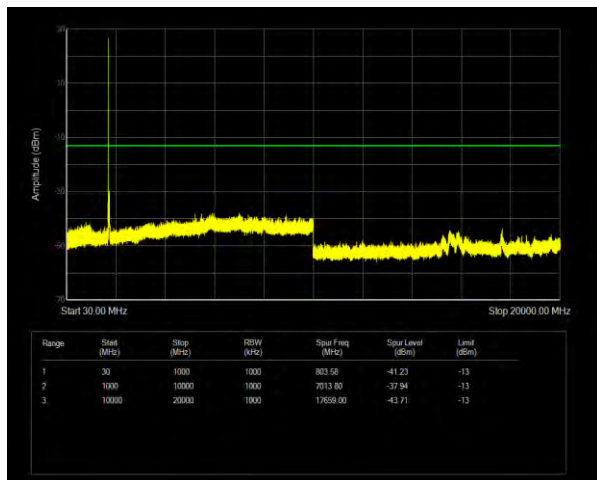
n66 SCS=15kHz DFT_BPSK BW=40MHz Channel=346000
