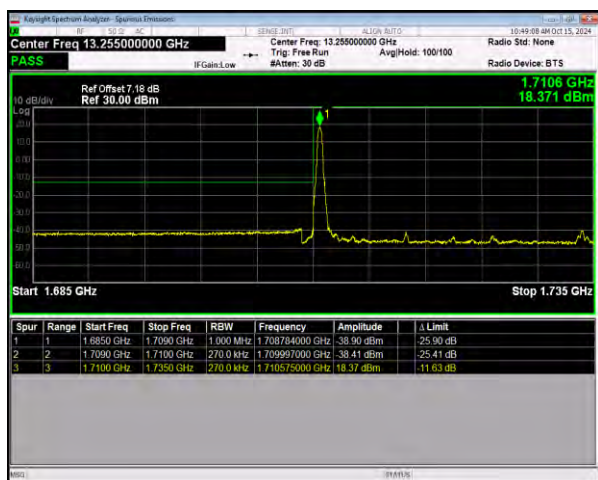
n66 SCS=15kHz DFT_256QAM BW=25MHz
