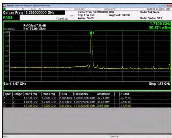
n66 SCS=15kHz DFT_64QAM BW=40MHz
