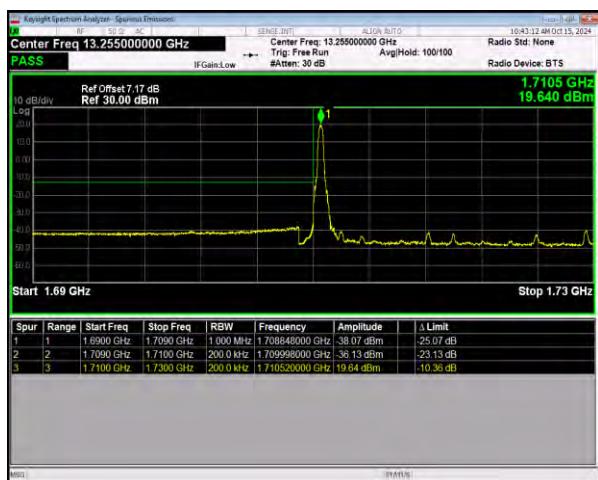
n66 SCS=15kHz DFT_64QAM BW=20MHz
