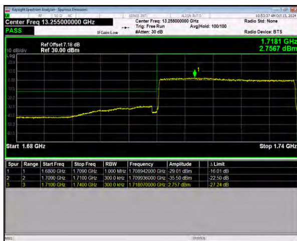
n66 SCS=15kHz DFT_16QAM BW=30MHz
