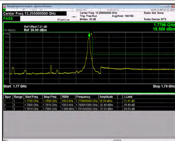
n66 SCS=15kHz DFT_QPSK BW=10MHz HighChannel=355000
