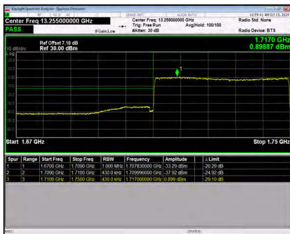
n66 SCS=15kHz DFT_256QAM BW=40MHz
