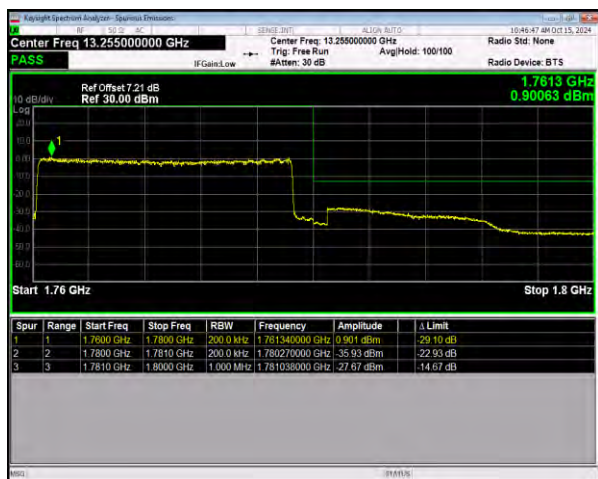
n66 SCS=15kHz DFT_256QAM BW=20MHz
