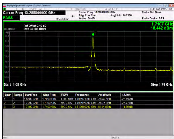
n66 SCS=15kHz DFT_256QAM BW=30MHz
