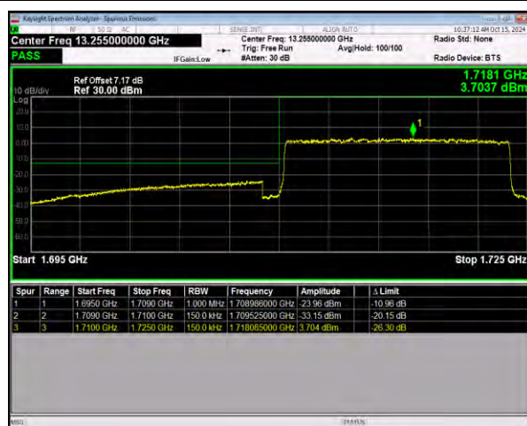
n66 SCS=15kHz DFT_QPSK BW=15MHz LowChannel=343500 RB=75@0
