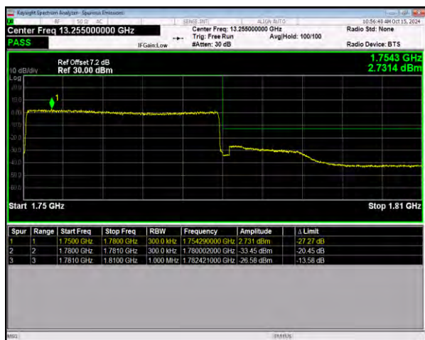
n66 SCS=15kHz DFT_64QAM BW=30MHz
