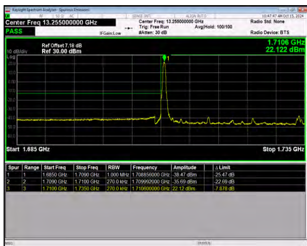
n66 SCS=15kHz DFT_QPSK BW=25MHz LowChannel=344500 RB=1@0
