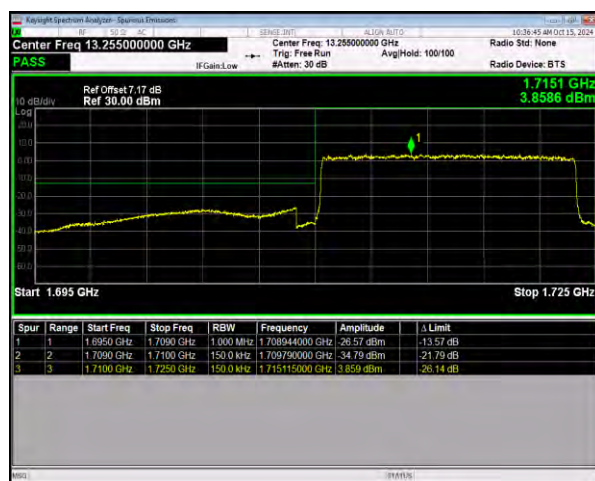
n66 SCS=15kHz DFT_BPSK BW=15MHz LowChannel=343500 RB=75@0
