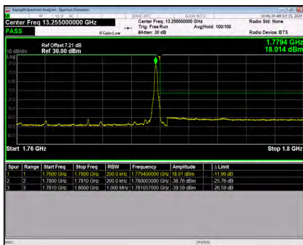
n66 SCS=15kHz DFT_256QAM BW=20MHz
