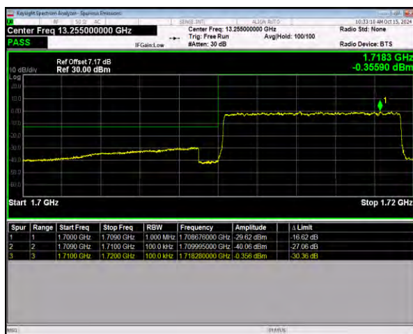
n66 SCS=15kHz DFT_256QAM BW=10MHz
