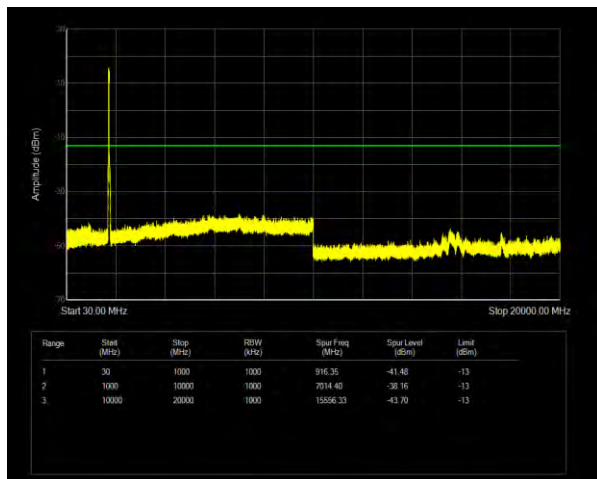
n66 SCS=15kHz DFT_BPSK BW=40MHz Channel=346000
