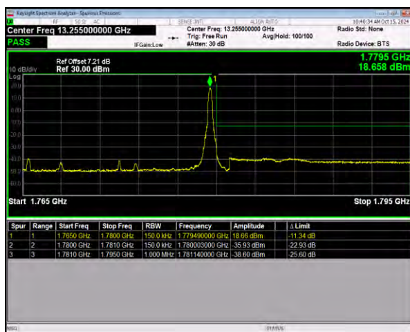
n66 SCS=15kHz DFT_64QAM BW=15MHz
