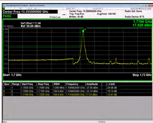
n66 SCS=15kHz DFT_64QAM BW=10MHz LowChannel=343000 RB=1@0
