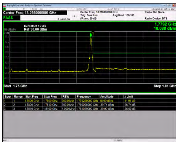
n66 SCS=15kHz DFT_256QAM BW=30MHz
