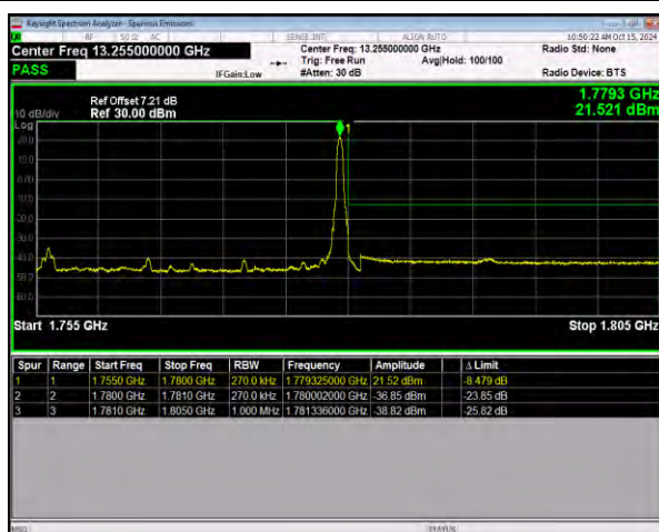
n66 SCS=15kHz DFT_QPSK BW=25MHz HighChannel=353500
