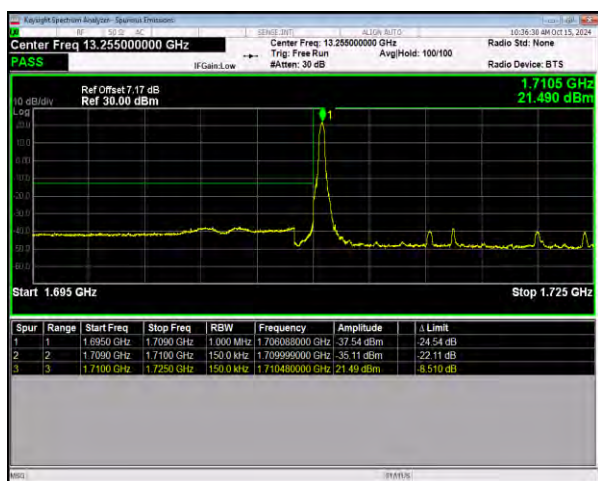
n66 SCS=15kHz DFT_BPSK BW=15MHz LowChannel=343500 RB=1@0
