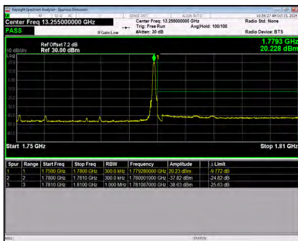
n66 SCS=15kHz DFT_64QAM BW=30MHz
