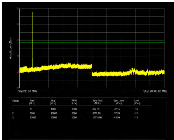
n66 SCS=15kHz DFT_BPSK BW=40MHz Channel=352000 RB=1@215
