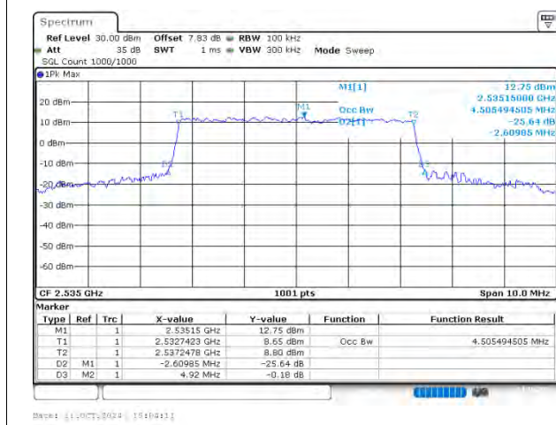
n7 SCS=15kHz CP_16QAM BW=5MHz Channel=507000 RB=25@0
