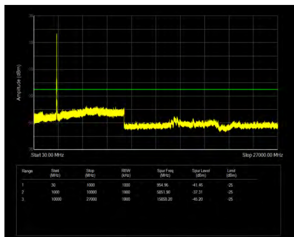
n7 SCS=15kHz DFT_BPSK BW=20MHz Channel=507000 RB=100@105
