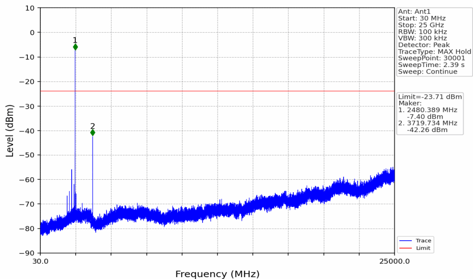
2M_HCH_2480MHz_Ant1_NTNV
