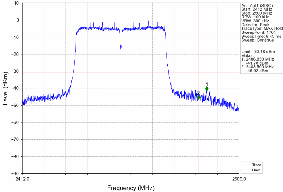
802.11n(HT40)_HCH_2452MHz_Ant1 (SISO)_NTNV
