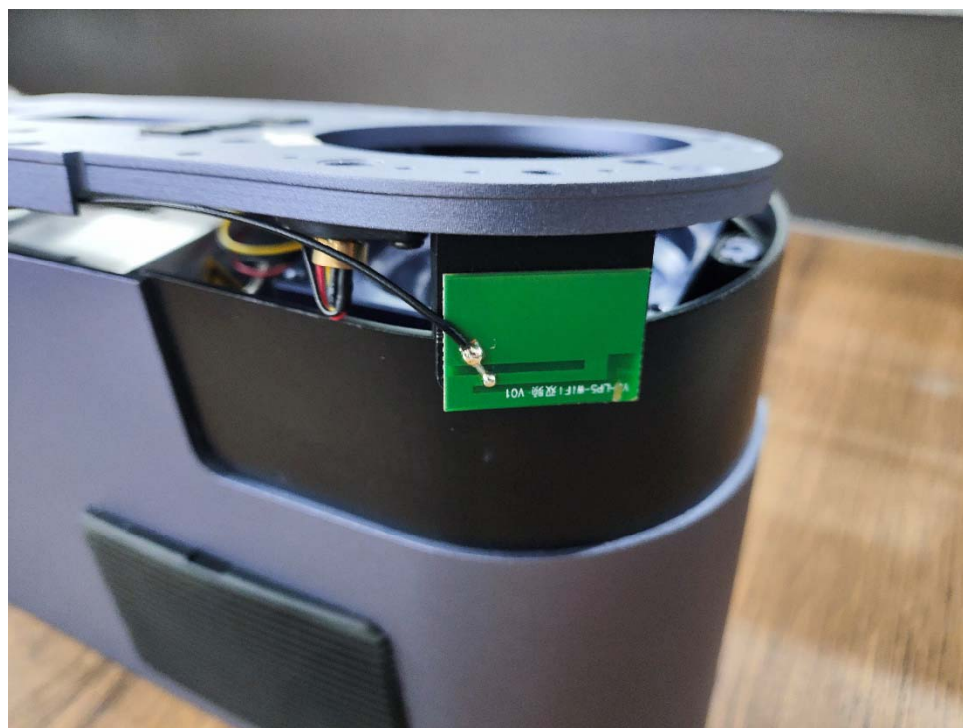
2.4G Antenna
