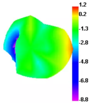
2500.000MHz E1
