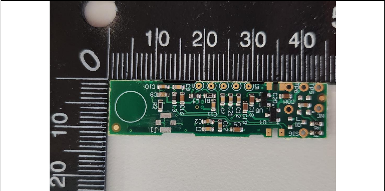
Bottom of EUT
