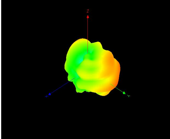
5150MHz
