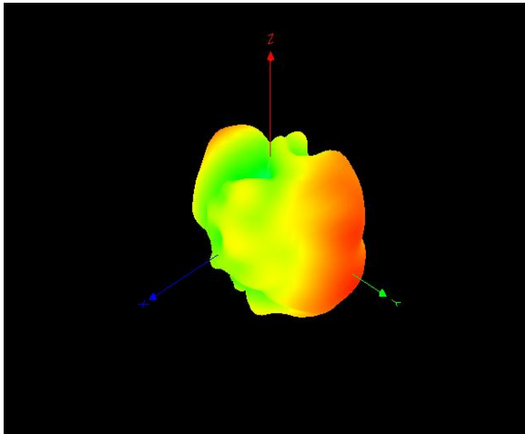
5850MHz
