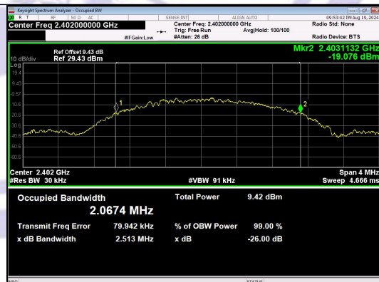
BLE 2M_Channel 0
