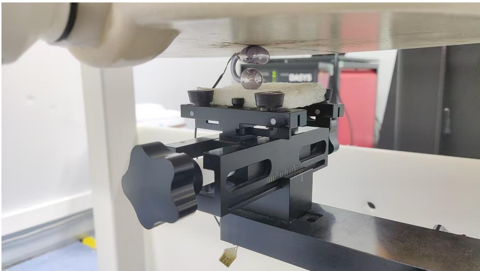
Right Edge (0mm)
