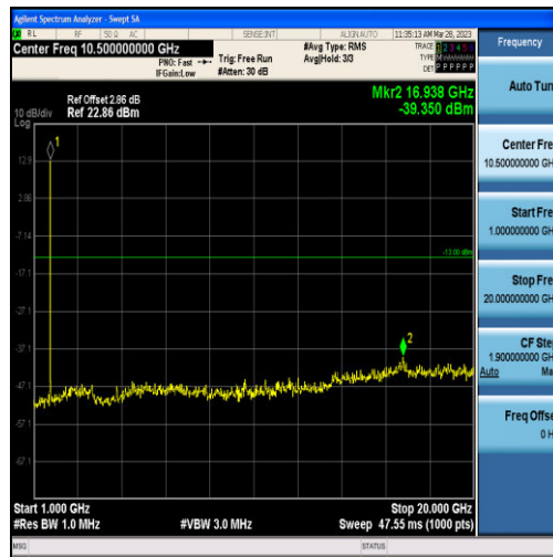
Band4-10MHz-16QAM-20000-50RB#0-Range2:1000~20000MHz
