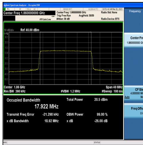
Band2-20MHz-QPSK-18700-100RB#0-17.922
