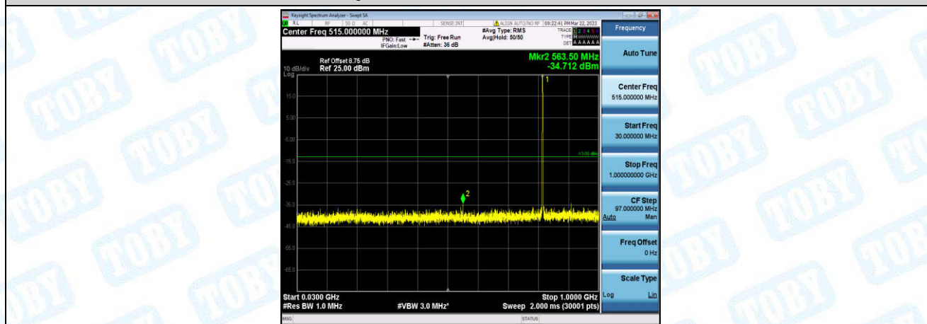
Band26-1.4MHz-16QAM-26740-1-0-Low-30-1000--34.71-PASS
