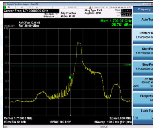
Band66-3MHz-QPSK-131987-1-0-Low--28.76-PASS
