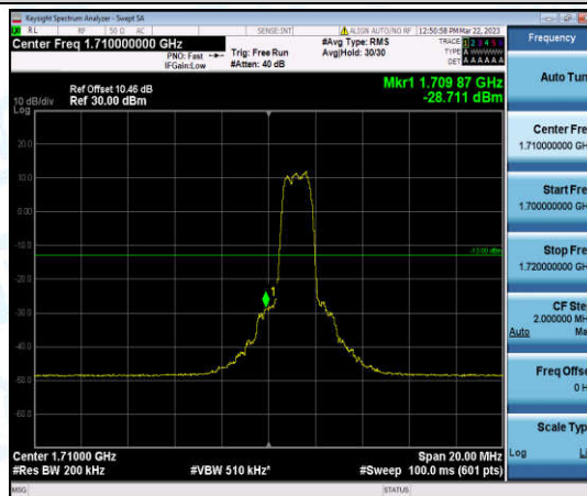
Band66-10MHz-QPSK-132022-6-0-Low--28.71-PASS
