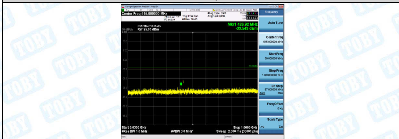
Band25-10MHz-QPSK-26090-1-0-Low-30-1000--33.54-PASS
