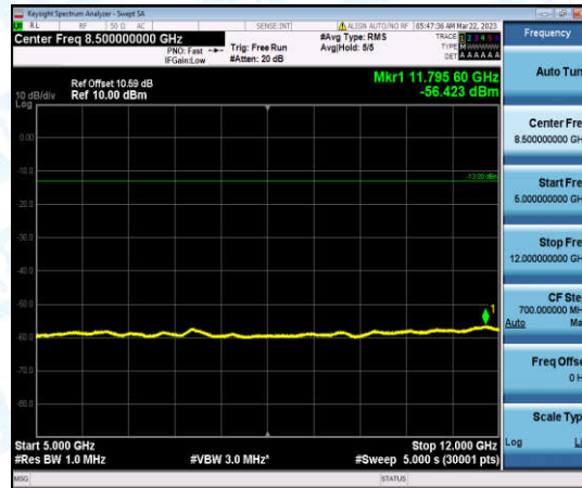
Band25-3MHz-QPSK-26365-1-0-Low-5000-12000--56.42-PASS
