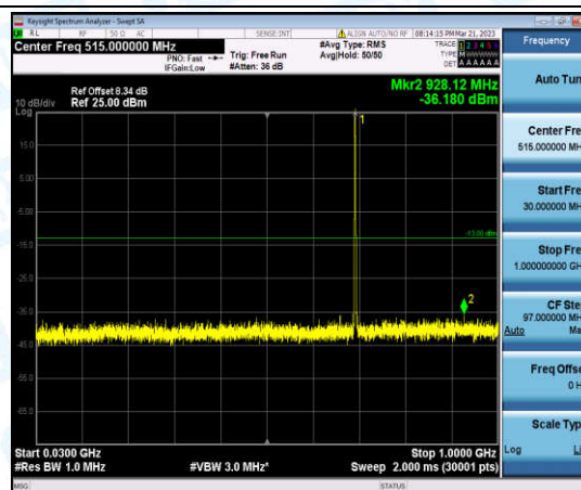
Band12-1.4MHz-QPSK-23017-1-0-Low-30-1000--36.18-PASS
