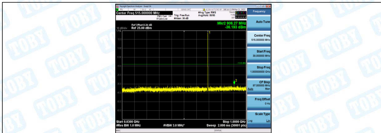
Band12-1.4MHz-16QAM-23017-1-0-Low-30-1000--36.19-PASS
