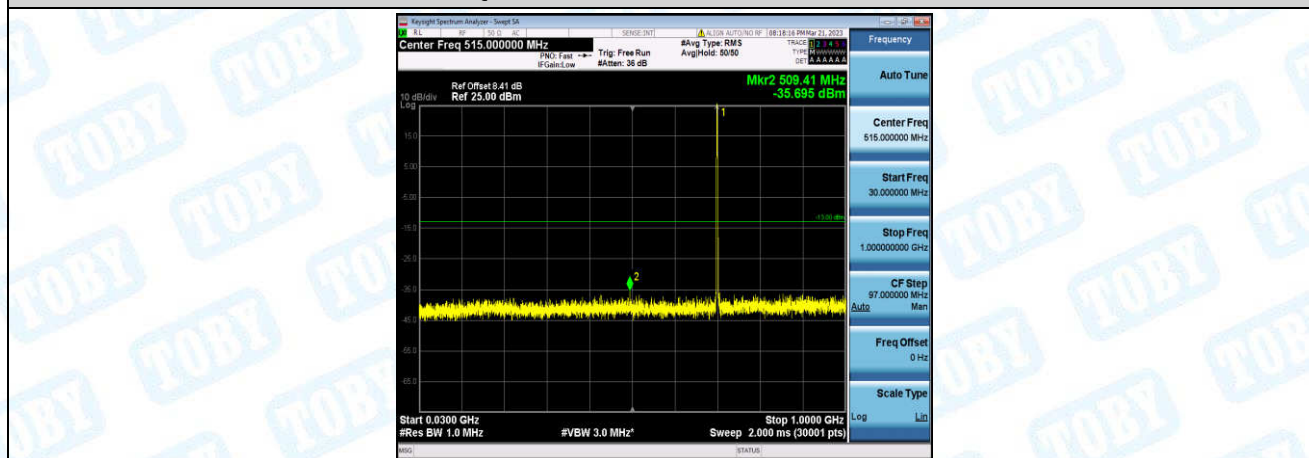
Band12-1.4MHz-QPSK-23095-1-0-Low-30-1000--35.7-PASS
