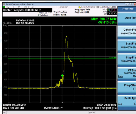
Band12-10MHz-16QAM-23060-1-0-Low--37.41-PASS
