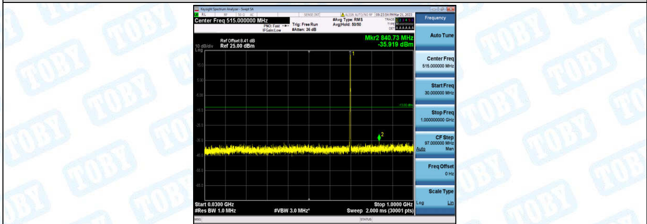
Band12-5MHz-16QAM-23095-1-0-Low-30-1000--35.92-PASS
