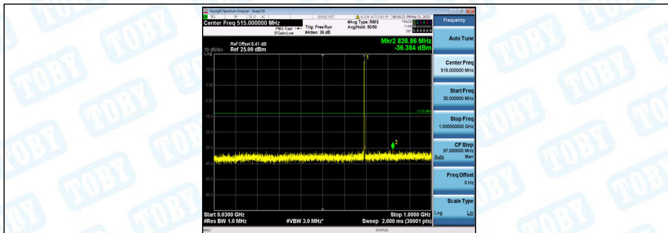
Band12-3MHz-QPSK-23025-1-0-Low-30-1000--36.38-PASS
