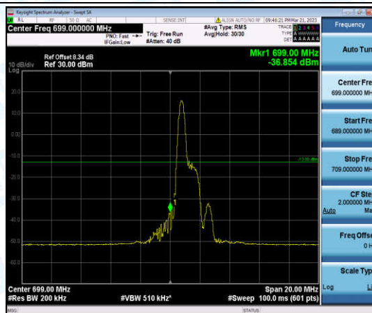
Band12-10MHz-QPSK-23060-1-0-Low--36.85-PASS
