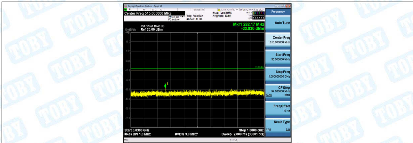
Band4-20MHz-QPSK-20050-1-0-Low-30-1000--33.83-PASS
